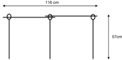
Type BPS 002
